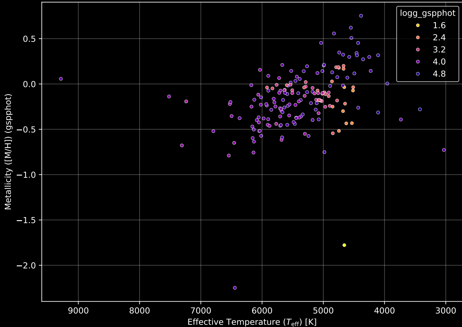
APOGEE DR17 Field: [263-30-O_TESS] Stellar Population Parameters (n= 174)
